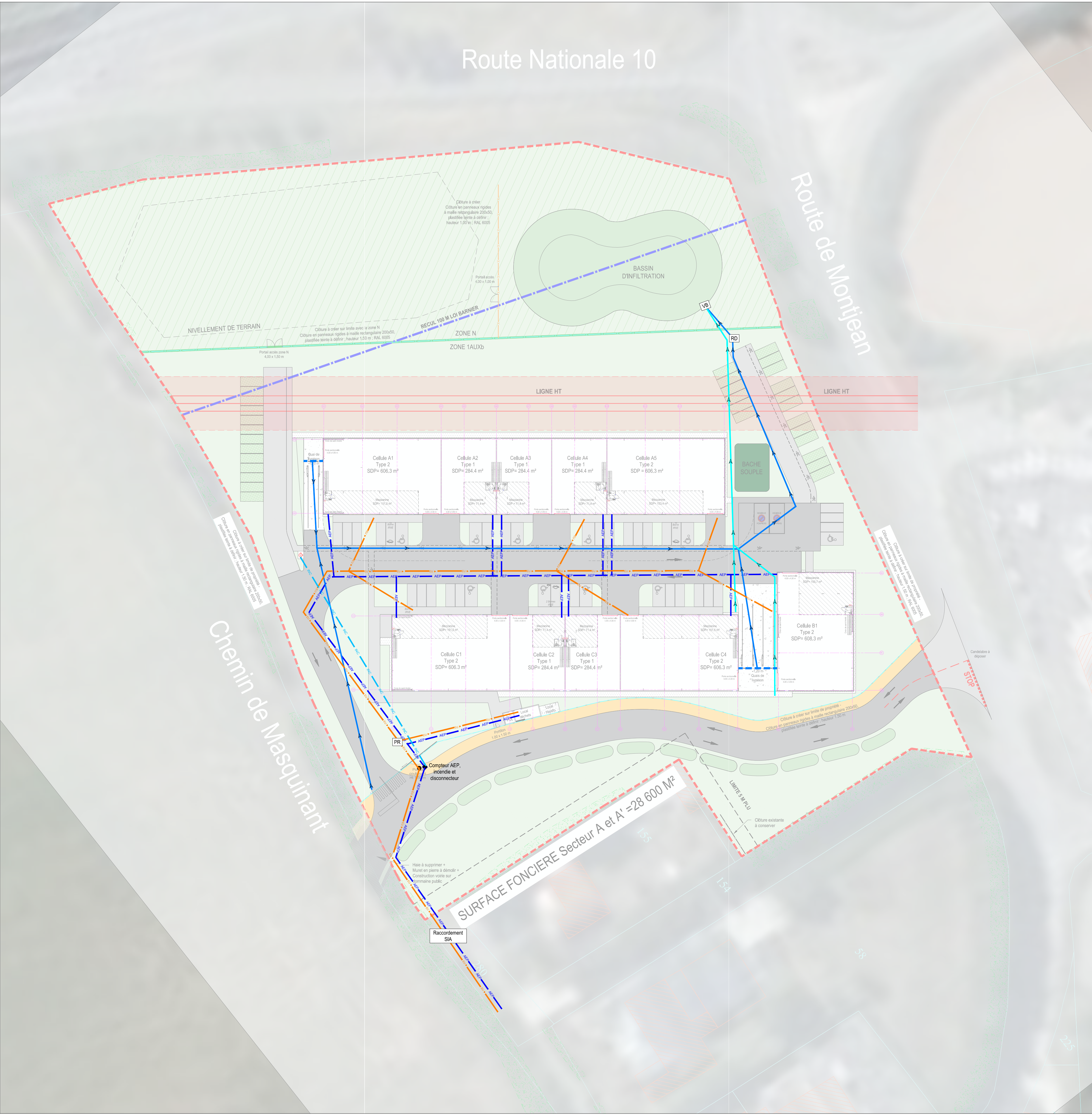
Plan repérage secteurs A - 1 : 2500
