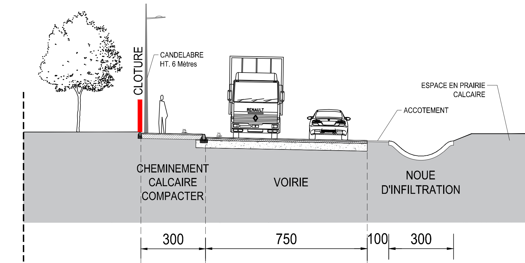
COUPES TN 3-3 - ECHELLE : 1-100
