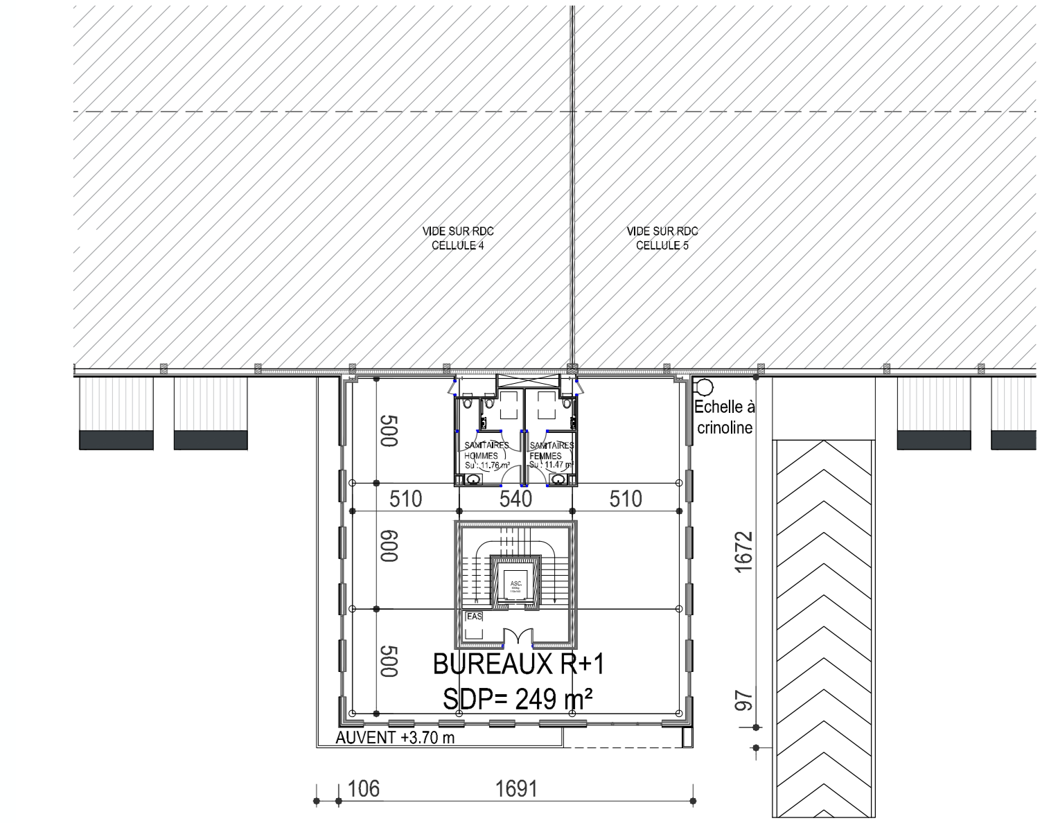
PLAN R+1 DES BUREAUX ENTRE CELLULE 4 ET 5 Echelle : 1/250
